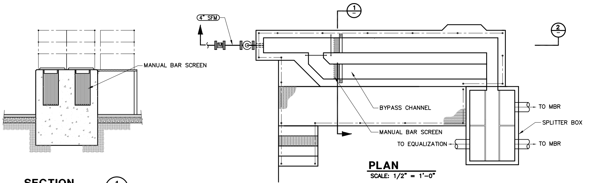
SECTION SCALE: 1/2" = 1'-0"
